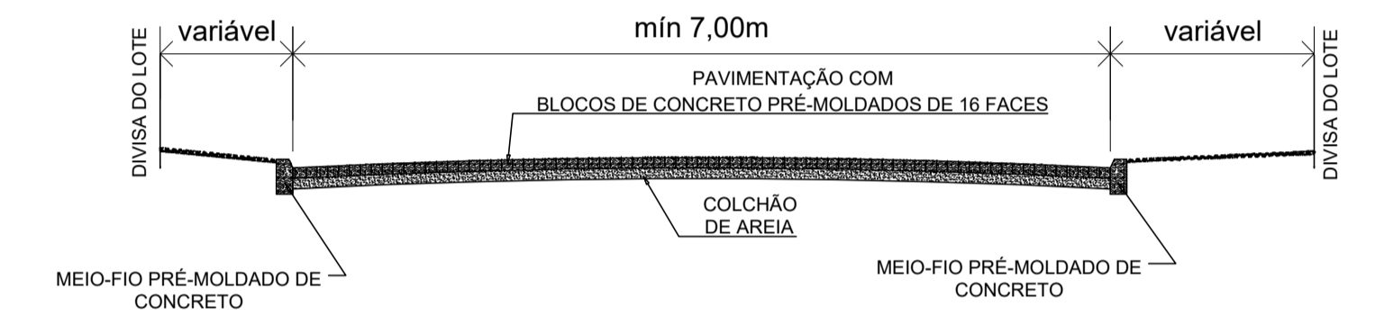
SEÇÃO TÍPICA DA PAVIMENTAÇÃO ESC 1:50
