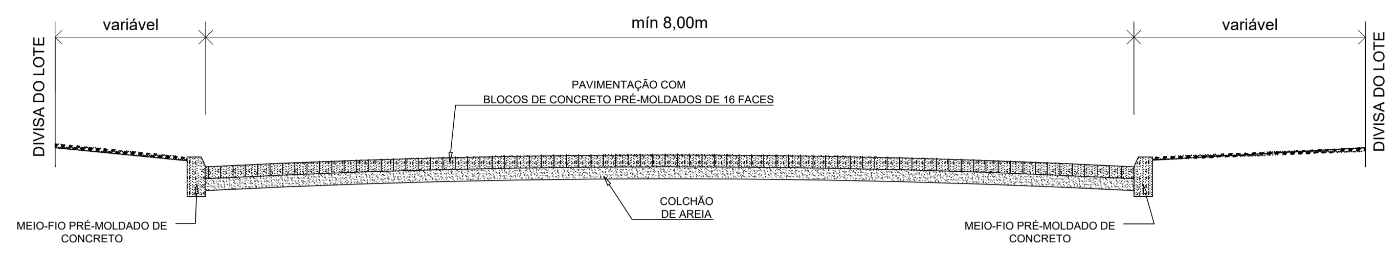
SEÇÃO TÍPICA DA PAVIMENTAÇÃO ESC 1:50
