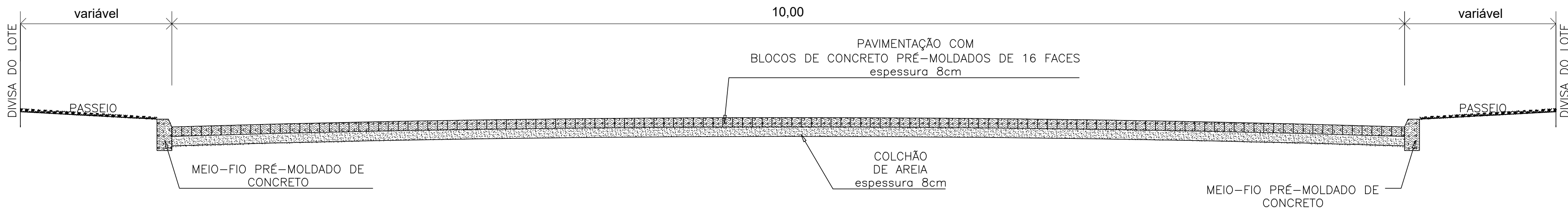
SEÇÃO TÍPICA PAVIMENTAÇÃO ESC 1:25
