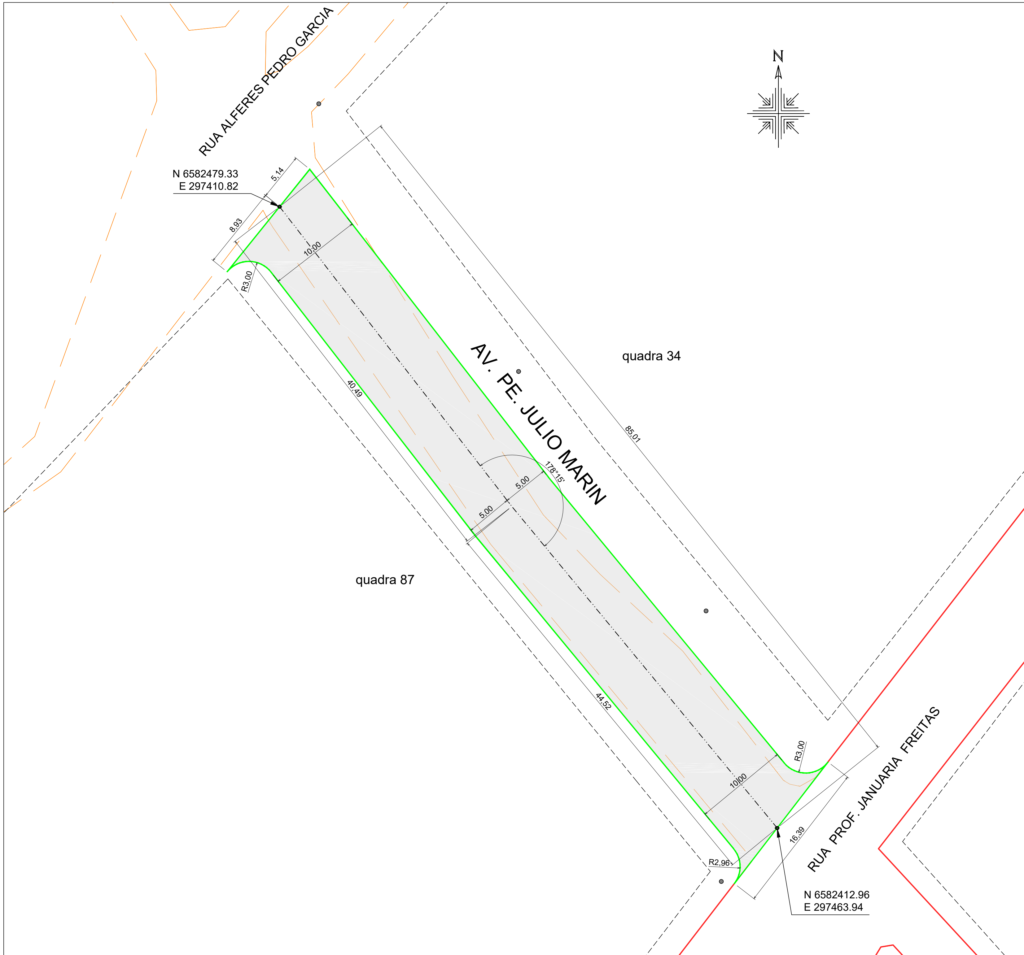
PLANTA-BAIXA ESC. 1:250
